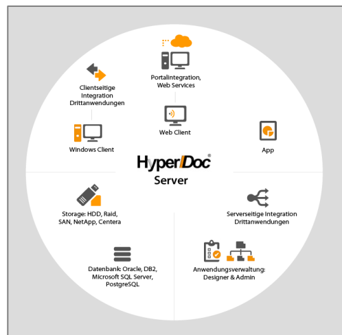
Abb. 2: HyperDoc Architektur
