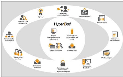
Abb. 1: Überblick HyperDoc
