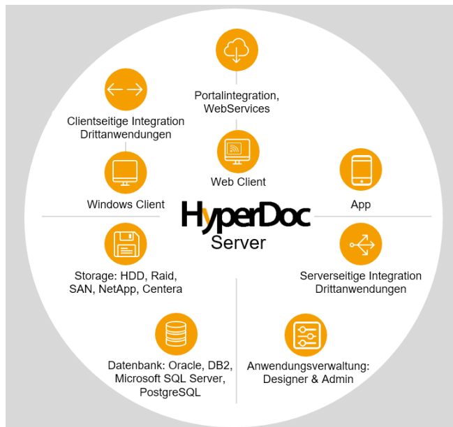
Abb.: Architektur HyperDoc
